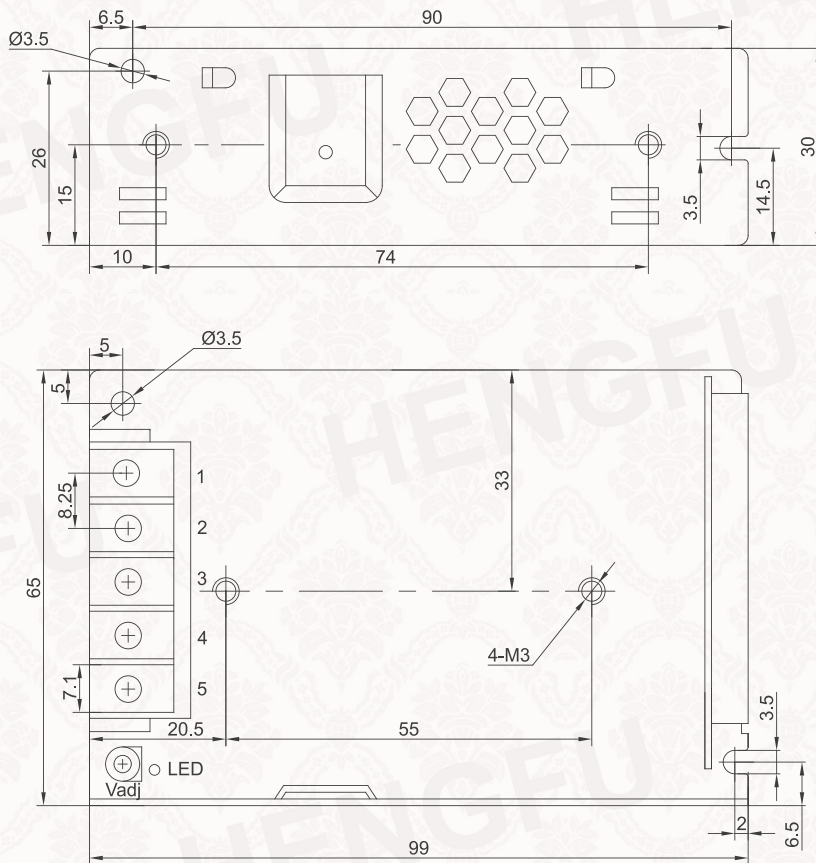
机壳 Frame
